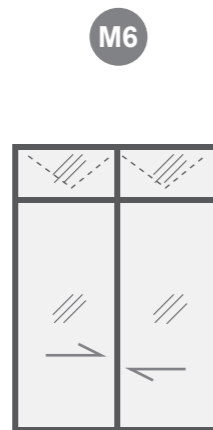
กว้าง 1.96 ม. สูง 2.60 ม. กระจกใส ด้านล่างเป็นบานสไลด์ ด้านบนเป็นบานกระทุ้ง + มุ้งลวด
