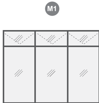
กว้าง 3.83 ม. สูง 2.60 ม. กระจกใส ด้านล่างเป็นบานตาย ด้านบนเป็นบานกระทุ้ง + มุ้งลวด
